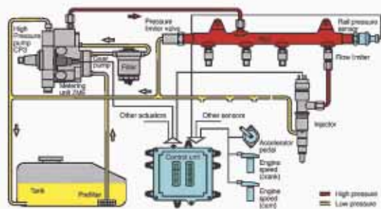
Motore "Common Rail" DOOSAN DL06
